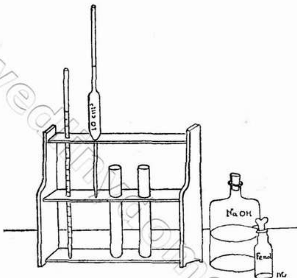
Ryc. 2. Najprostsze przybory do oznaczenia kwasowości.
