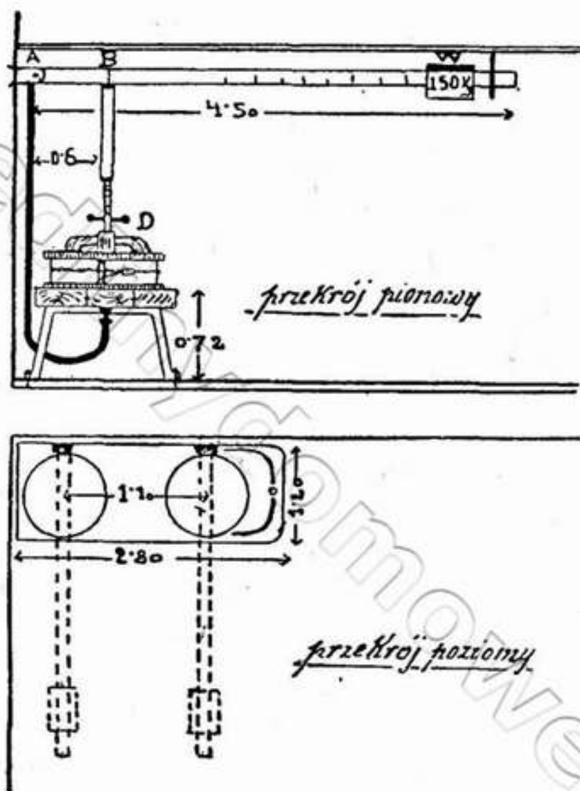
Ryc. 33. Prasa Schatzmanna.
