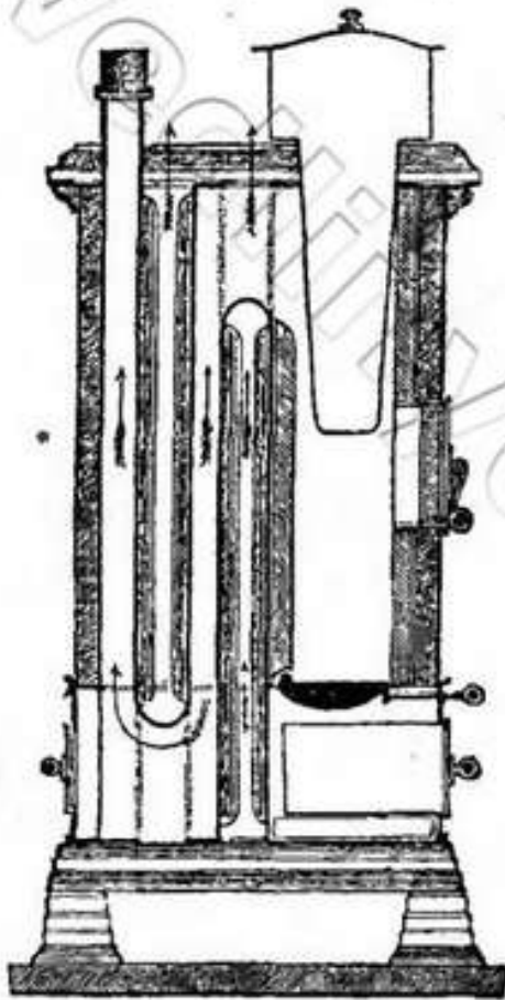
Pyc. 50. Przekrój pionowy pieca systemu Santé.
