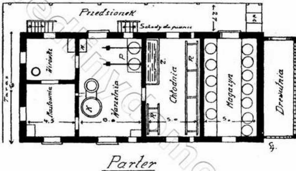
Ryc. 46. Rzut poziomy.
